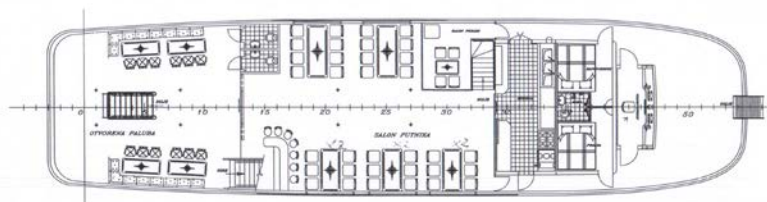
Hauptdeck
