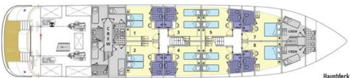
Hauptdeck
