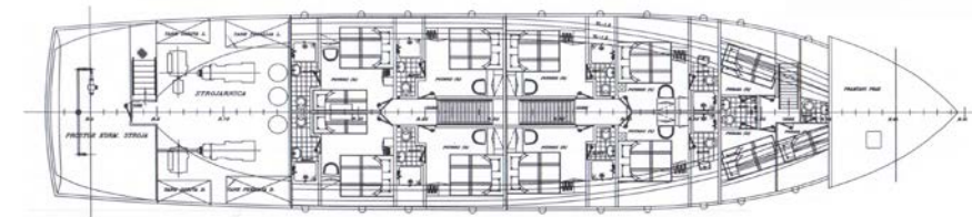
Kabinendeck
