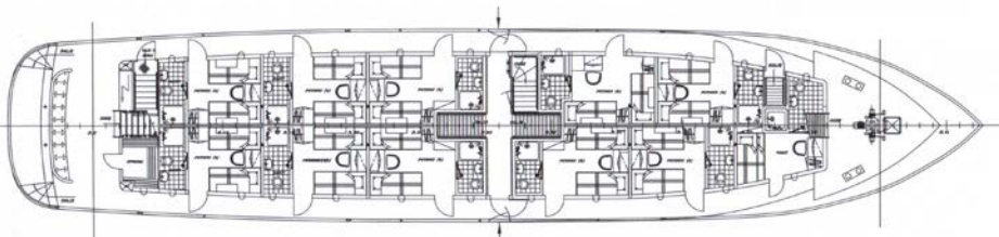
Kabinendeck
